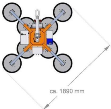
Přísavka WH800
